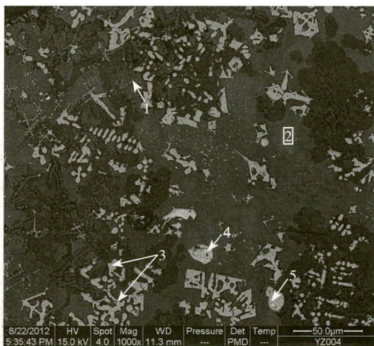
图三 汤家墩炉壁挂渣89T7⑤：9背散射电子像（EDS微区分析：1. 铜铁相 2. 铁氧化物 3、4. 纯铜颗粒）
