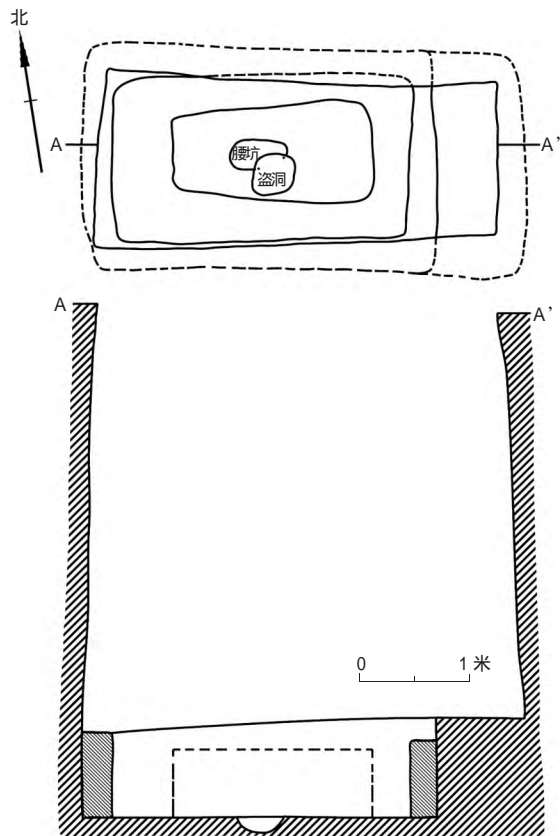
图四 2012SCXM1 平面图
