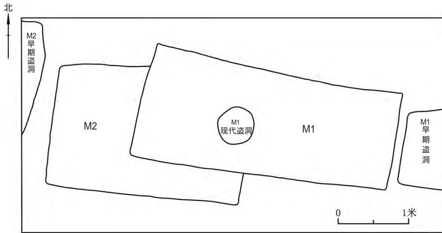
图三 2012SCXT1 平面图
